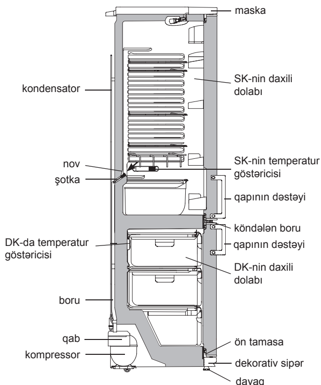
Şəkil 7 — SK-dən qar suyunun axma sistemi
